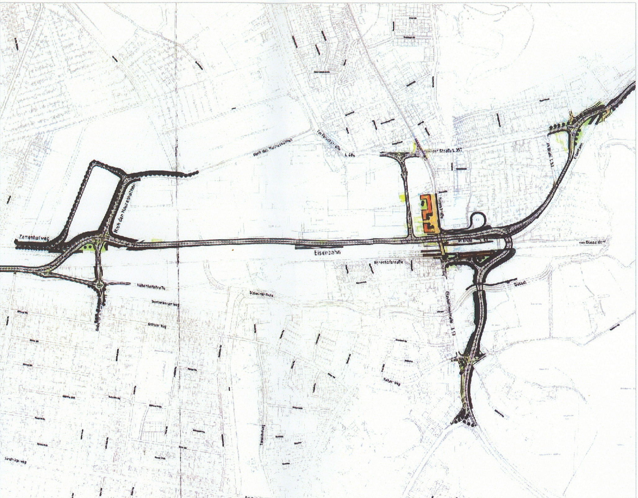
Abbildung 7: Geplanter Verlauf der L 404n – Auszug aus der Machbarkeitsstudie „L 404n – Umgehung Gerresheim von Ronsdorfer Straße bis Morper Straße / Vennhauser Allee“ (ohne Maßstab)
